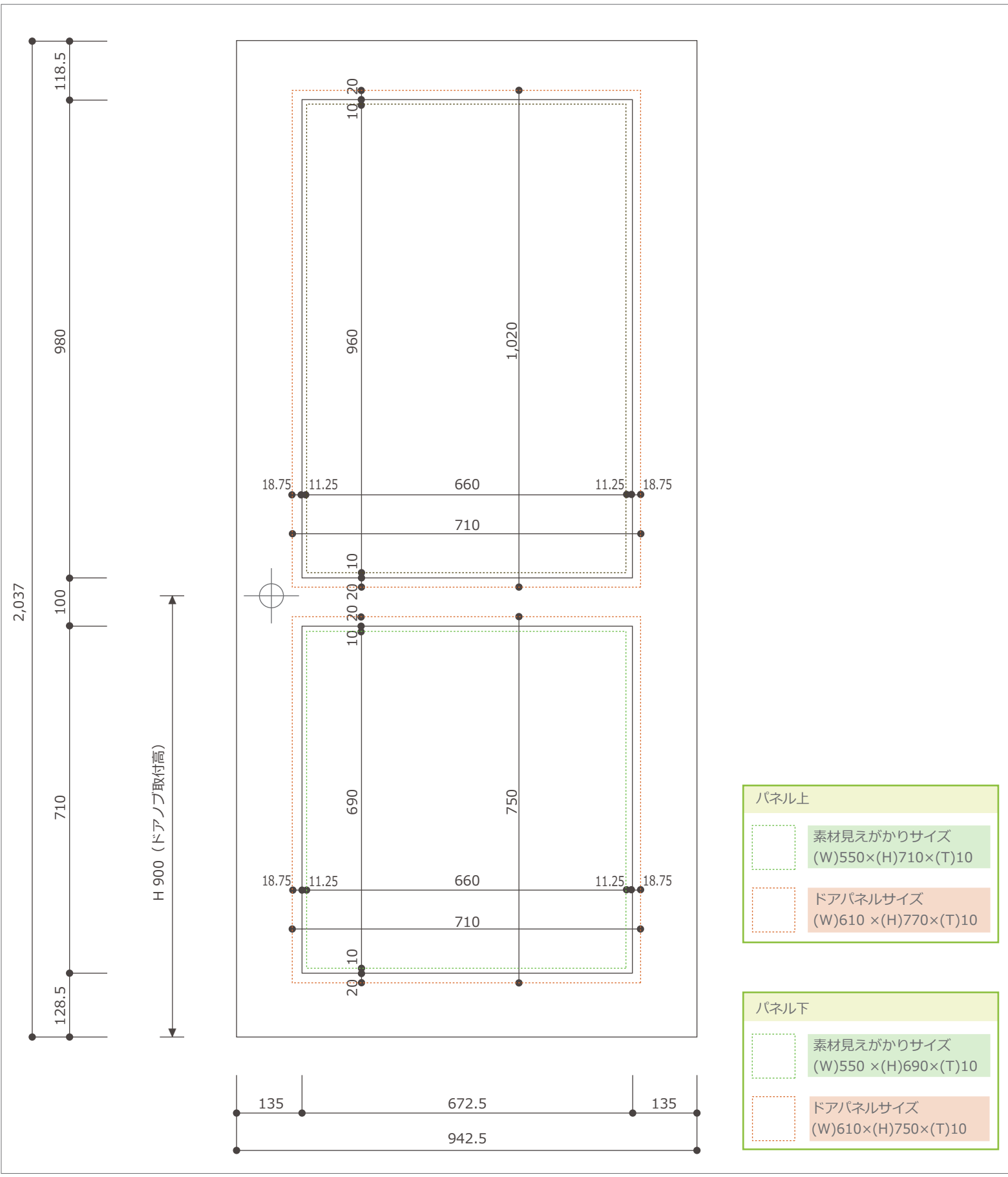
引き違い戸規格サイズ -2 (W)942.5 ×(H)2,037×(T)31
