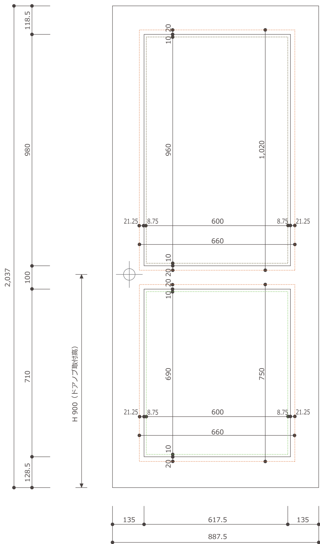
片引き戸規格サイズ-2 (W)887.5×(H)2,037×(T)33
