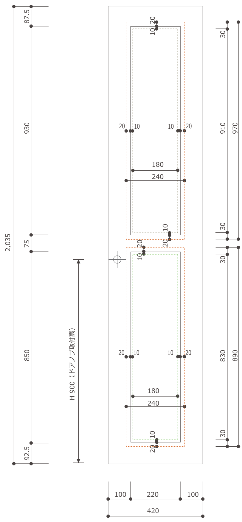
軸吊折戸規格サイズ-2 (W)420×(H)2,035×(T)30
